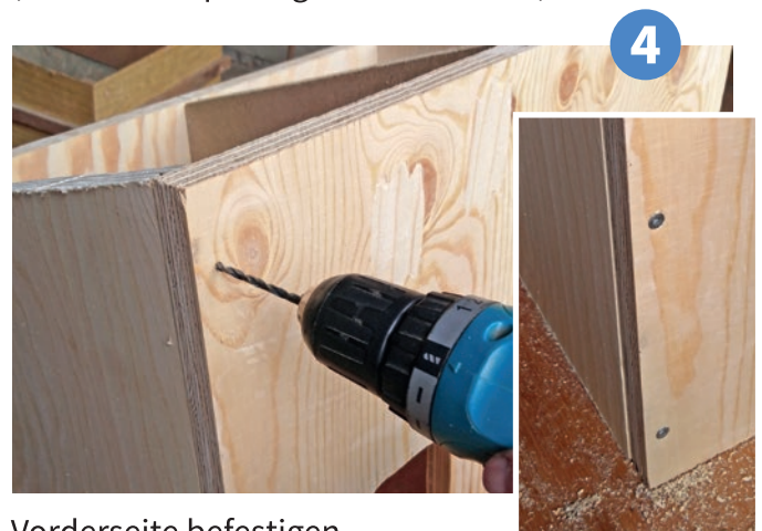
Vorderseite befestigen
